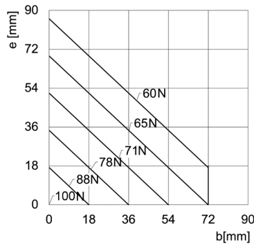
CGPT-25-NC apertura
