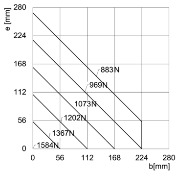
CGPT-80 apertura
