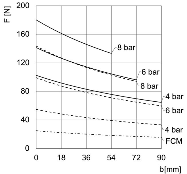
CGPT-25-NC
