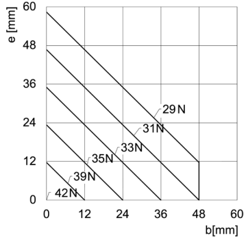
CGPT-16-NC apertura
