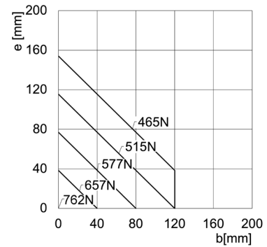
CGPT-50-NO apertura
