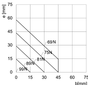
CGPT-20-NC chiusura
