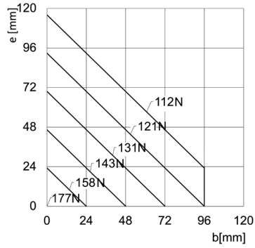
CGPT-32-NC apertura
