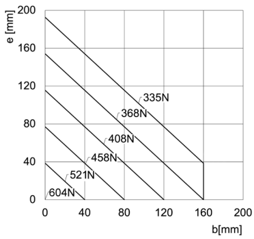
CGPT-50 apertura
