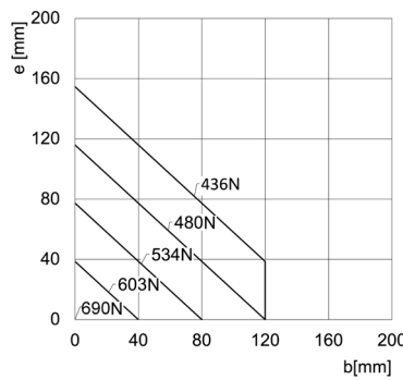
CGPT-50-NC chiusura
