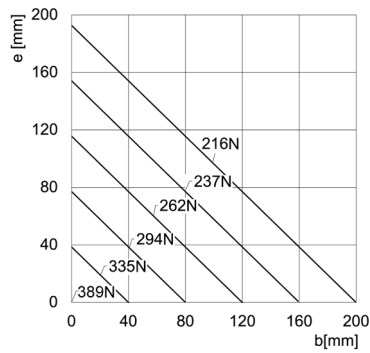
CGPT-50-NC apertura
