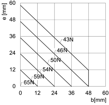
CGPT-16 apertura
