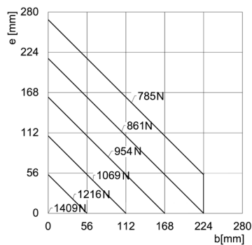
CGPT-80 chiusura
