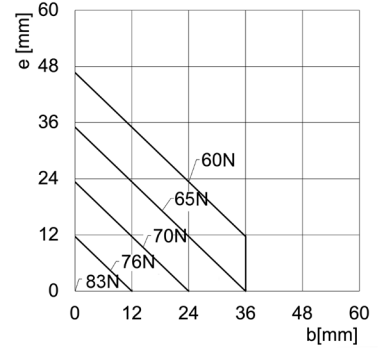
CGPT-16-NO apertura
