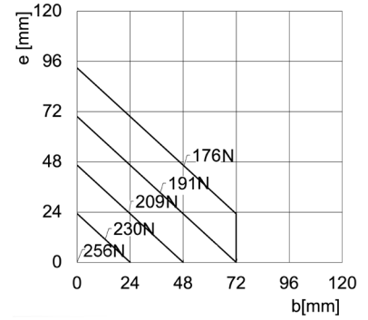
CGPT-32-NO apertura
