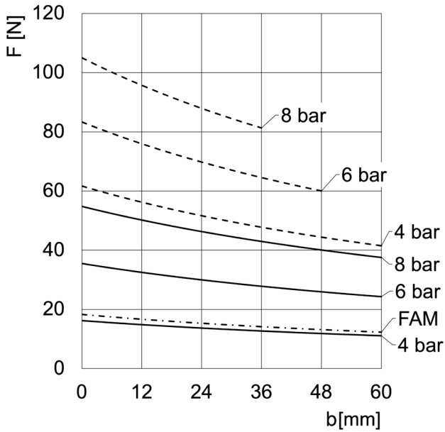
CGPT-16-NO
