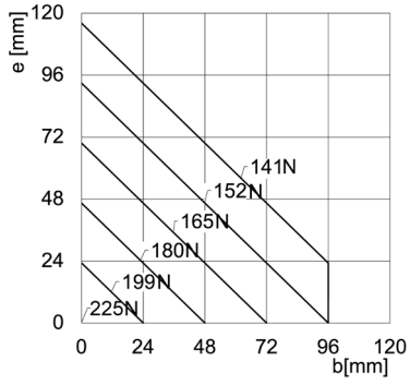
CGPT-32 apertura
