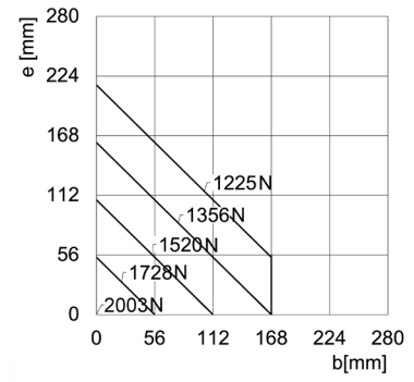
CGPT-80-NO apertura
