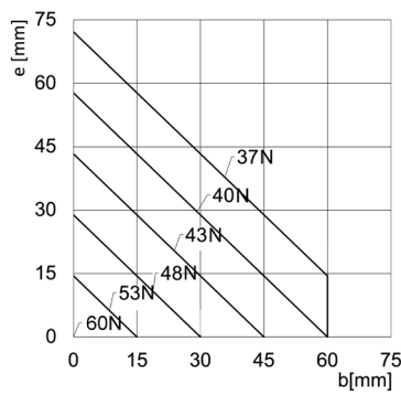
CGPT-20-NC apertura
