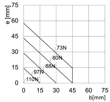
CGPT-20-NO apertura
