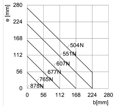
CGPT-80-NO chiusura
